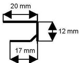
U-profil 10mm
