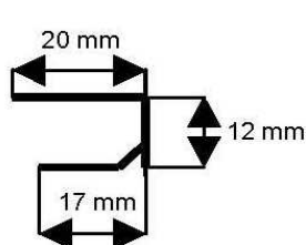
U-profil 10mm
